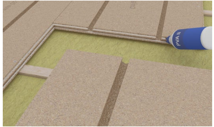
Figur 6 Påför rikligt med lim på regler och fjäderns båda ovsidor.
